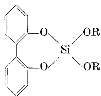
Di-natrium-bis-0,0'-diphenolato-bismethanolato-silikat
