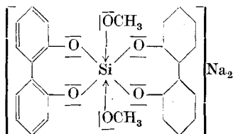
Di-natrium-bis-0,0'-diphenolato-bismethanolato-silikat
